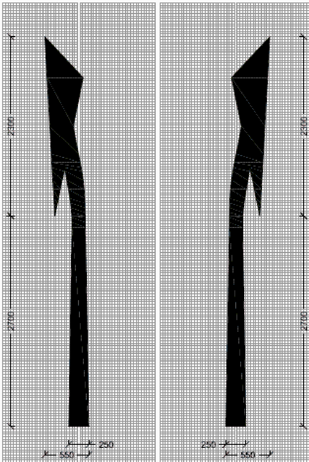
ΒΑΛΛΑ : αλλαγή λωρίδας προς αριστερά ΒΑΛΔ : αλλαγή λωρίδας προς δεξιά
