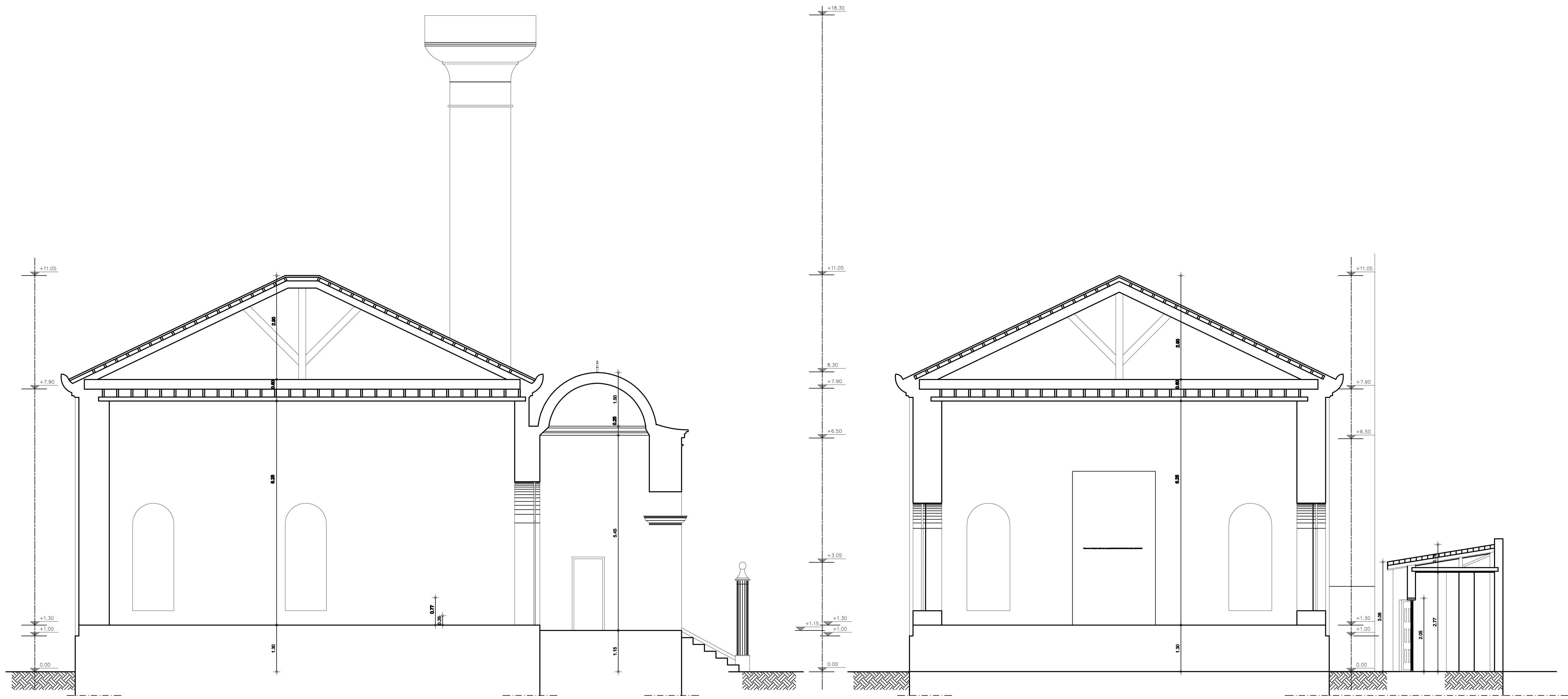
ΤΟΜΗ Β-Β
