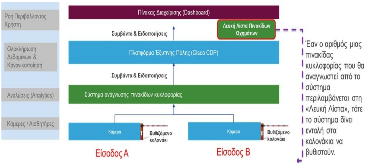
Αρχιτεκτονικό διάγραμμα διασύνδεσης τμημάτων λογισμικού
